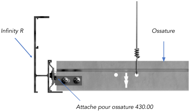
Infinity R sur ossature de plafond suspendu
