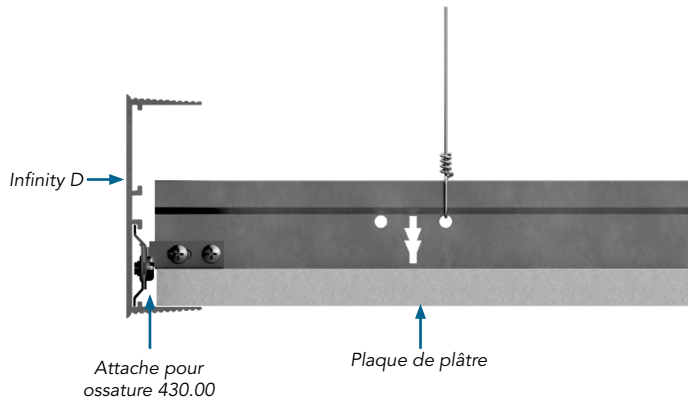
Installation de moulure Infinity avec ossature pour plaques de plâtre
