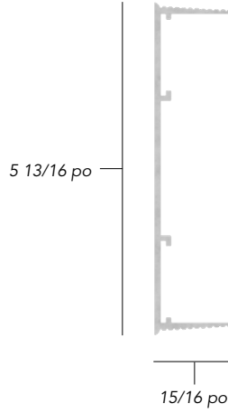
Moulure Infinity D de 6 po
