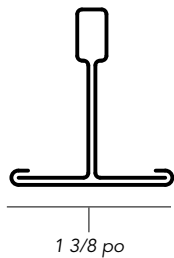
Ossature pour plaques de plâtre 640/650
