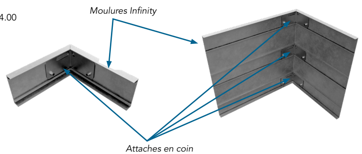
Installation d'attaches en coin
