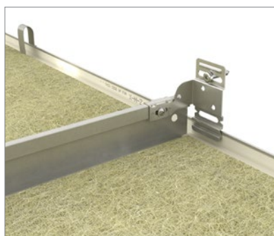
Om de haaksheid van het systeem te waarborgen, wordt geadviseerd om elk hoofdprofiel en elk tweede tussenprofiel aan de wand te bevestigen middels een 90° beugel.
